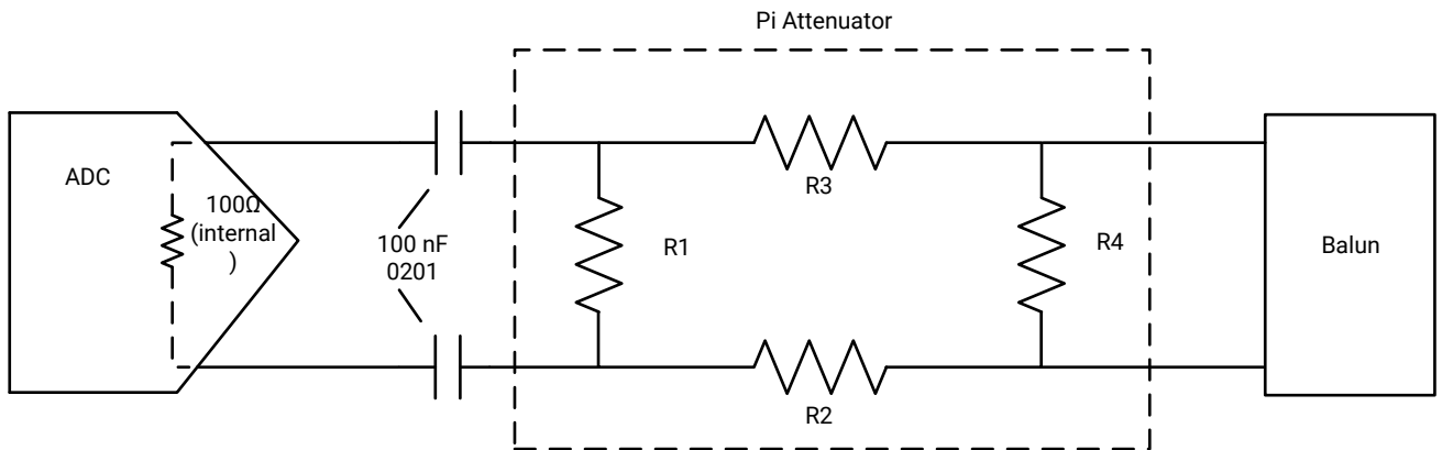
Figure 135: -2 dB Pi Attenuation Network (XCZU25DR/XCZU27DR/XCZU28DR/XCZU29DR)
