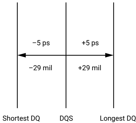
Figure 12: Skew Example for DQ to DQS
